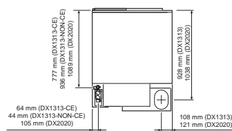
Seitenansicht DX 13/13 20/20 Gas
