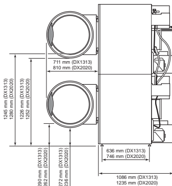
Seitenansicht DX 13/13 20/20
