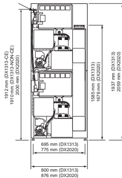
Seitenansicht DX 13/13 20/20 Gas
