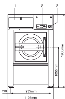
FRONTANSICHT FS 33 40 55
