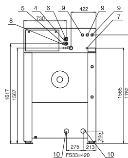
RÜCKANSICHT FS 33 40 55
